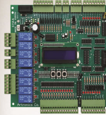
كارت ارت رونيك (مصري) Artronic Card (EG)
