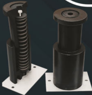
سوستة بئر Pit Spring
